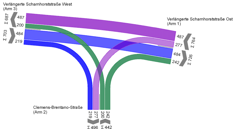
Abbildung 8-20: KP4 Verlängerte Scharnhorststraße/Clemens-Brentano Straße, DTV 2030, Var A
