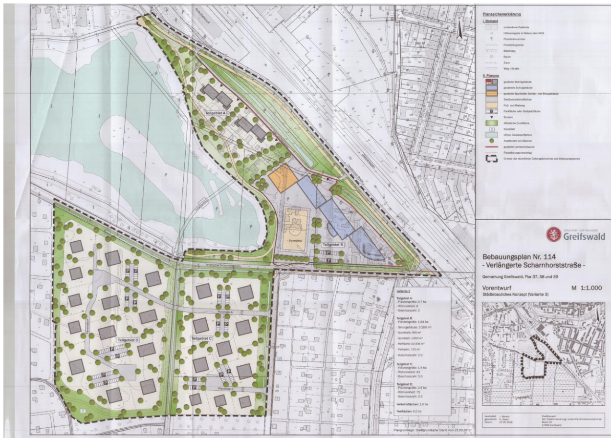
Abbildung 1-2: B-Plan Vorentwurf (Variante 3) Stand Mai 2018 zu Beginn der hydrologischen Studie (Quelle: Stadtplanungsamt Greifswald)
