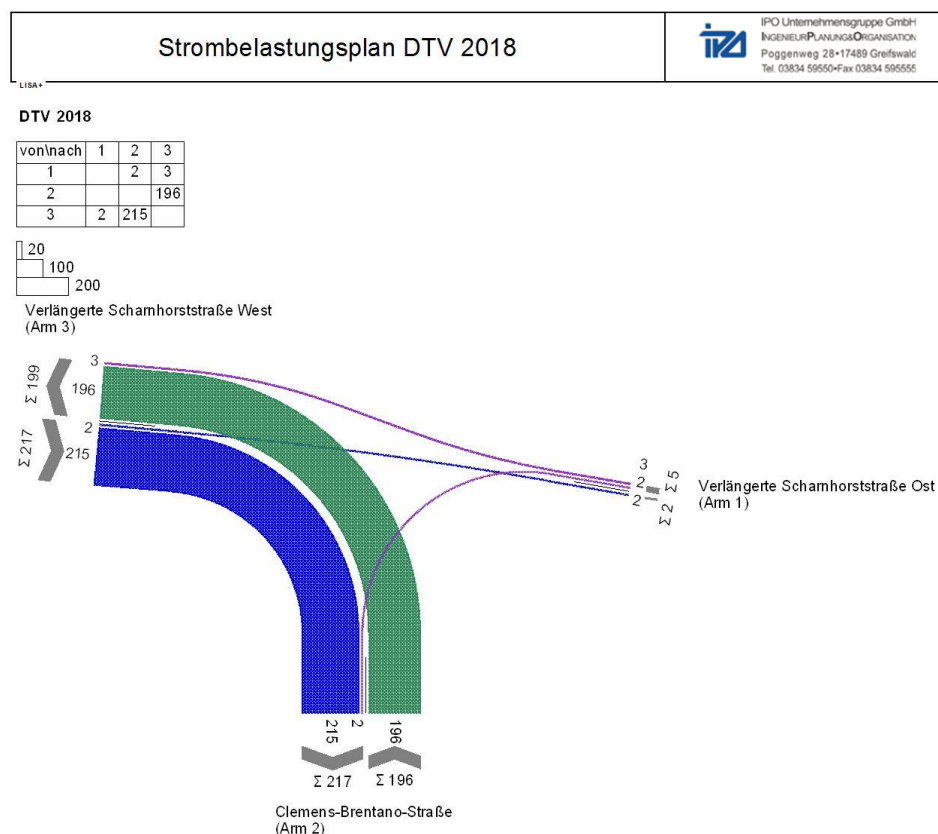
Abbildung 8 KP4 Verlängerte Scharnhorststraße/Clemens-Brentano Straße, DTV 2018
