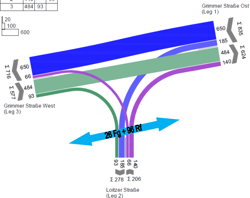
Abbildung 8-17: KP3, Vor- und Nachmittagsspitzenstunde 2030 Var C
