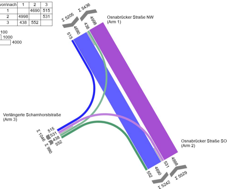
Abbildung 8-4: KP1 Osnabrücker Straße/Verlängerte Scharnhorststraße, DTV 2030- Var B
