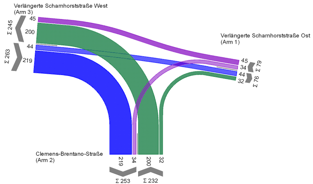
Abbildung 8-24: KP4 Verlängerte Scharnhorststraße/Clemens-Brentano Straße, DTV 2030, Var C.
