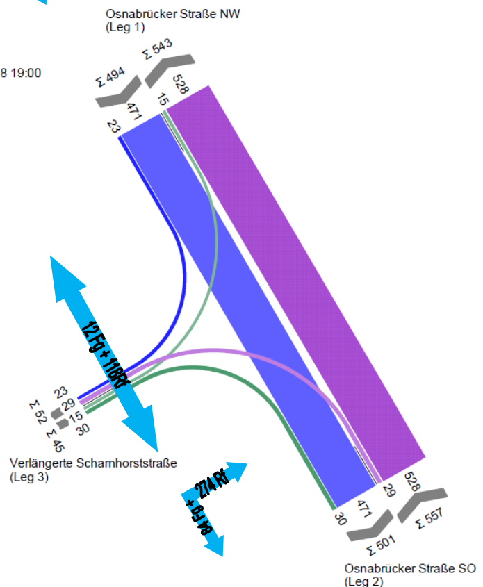
Abbildung 8-3: KP1, Vor- und Nachmittagsspitzenstunde 2030 Var B
