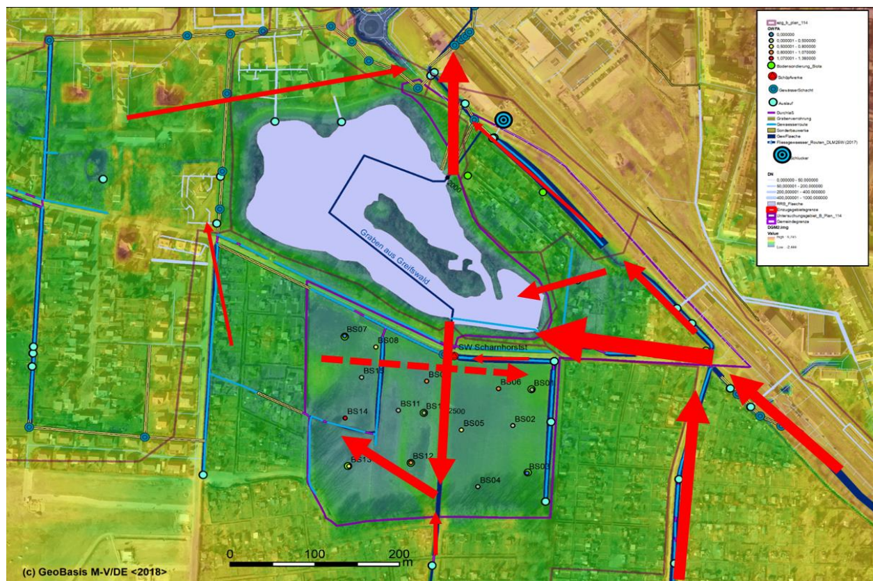
Abbildung 3-30: Fließverhalten der Gewässer im HQ-100-Fall mit Umkehrung der Fließrichtung am Graben 25 oberhalb des RRB
