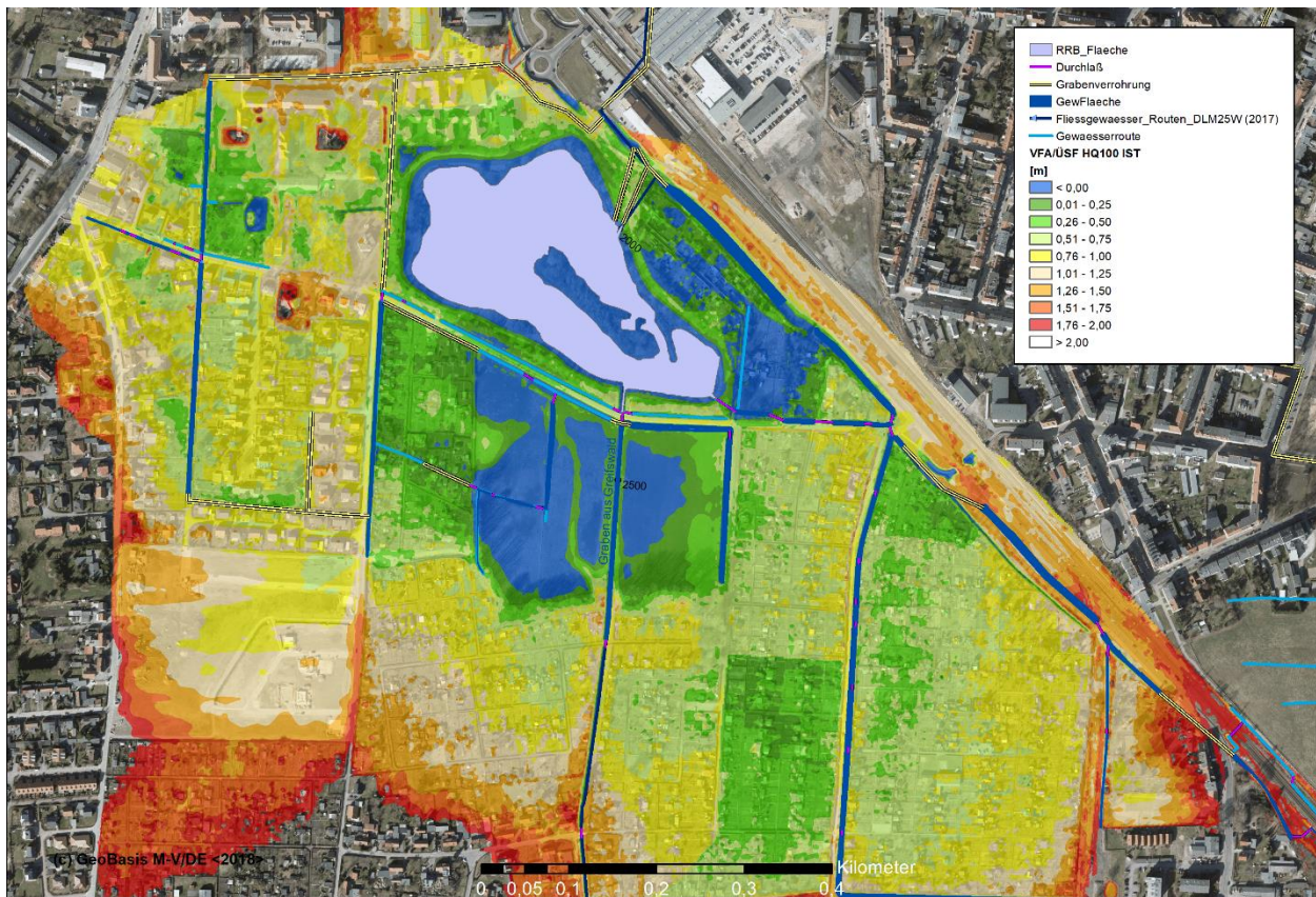
Abbildung 3-31: Vorflutabstände (grün-rot) / Überschwemmungsflächen (blau) bei HQ 100 im IST-Zustand
