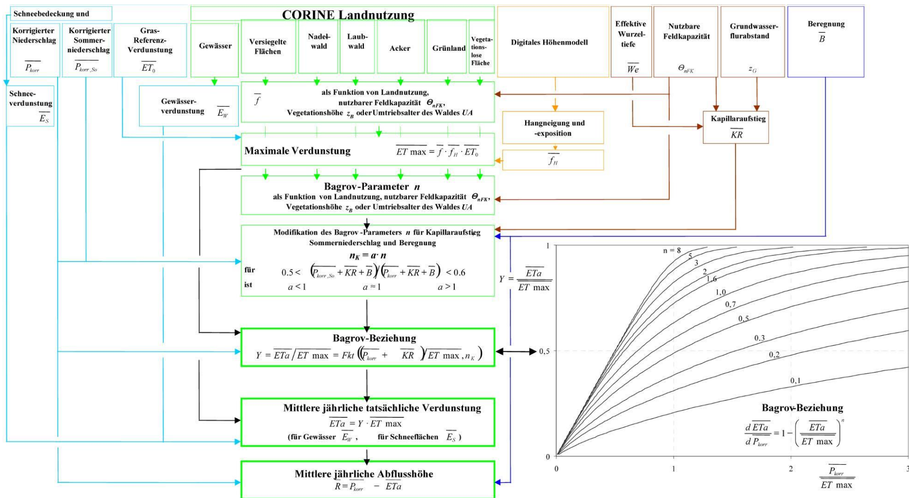
Abbildung 3-9: Schema zur Berechnung der mittleren jährlichen tatsächlichen Verdunstung und des mittleren Gesamtabflusses nach dem Wasserhaushaltsverfahren BAGLUA (GLUGLA et al. 1999) (Quelle: BFG 2003)
