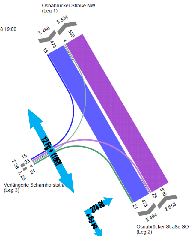
Abbildung 8-1: KP1, Vor- und Nachmittagsspitzenstunde 2030 Var A
