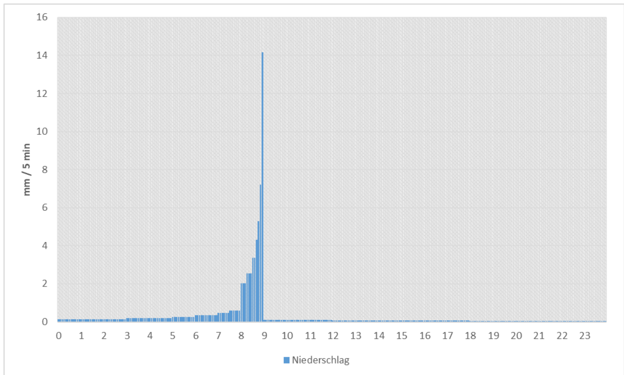
Abbildung 3-27: Angewendete Niederschlagsverteilung KOSTRA-EULER-II
