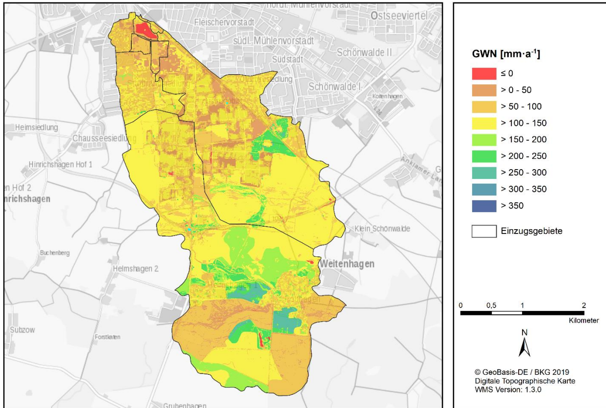
Abbildung 3-21: Mittlere jährliche Grundwasserneubildungshöhe nach BAGLUVA und MEIER (2013) für die Dekaden 1981-2010 im Untersuchungsgebiet (IST-Zustand)
