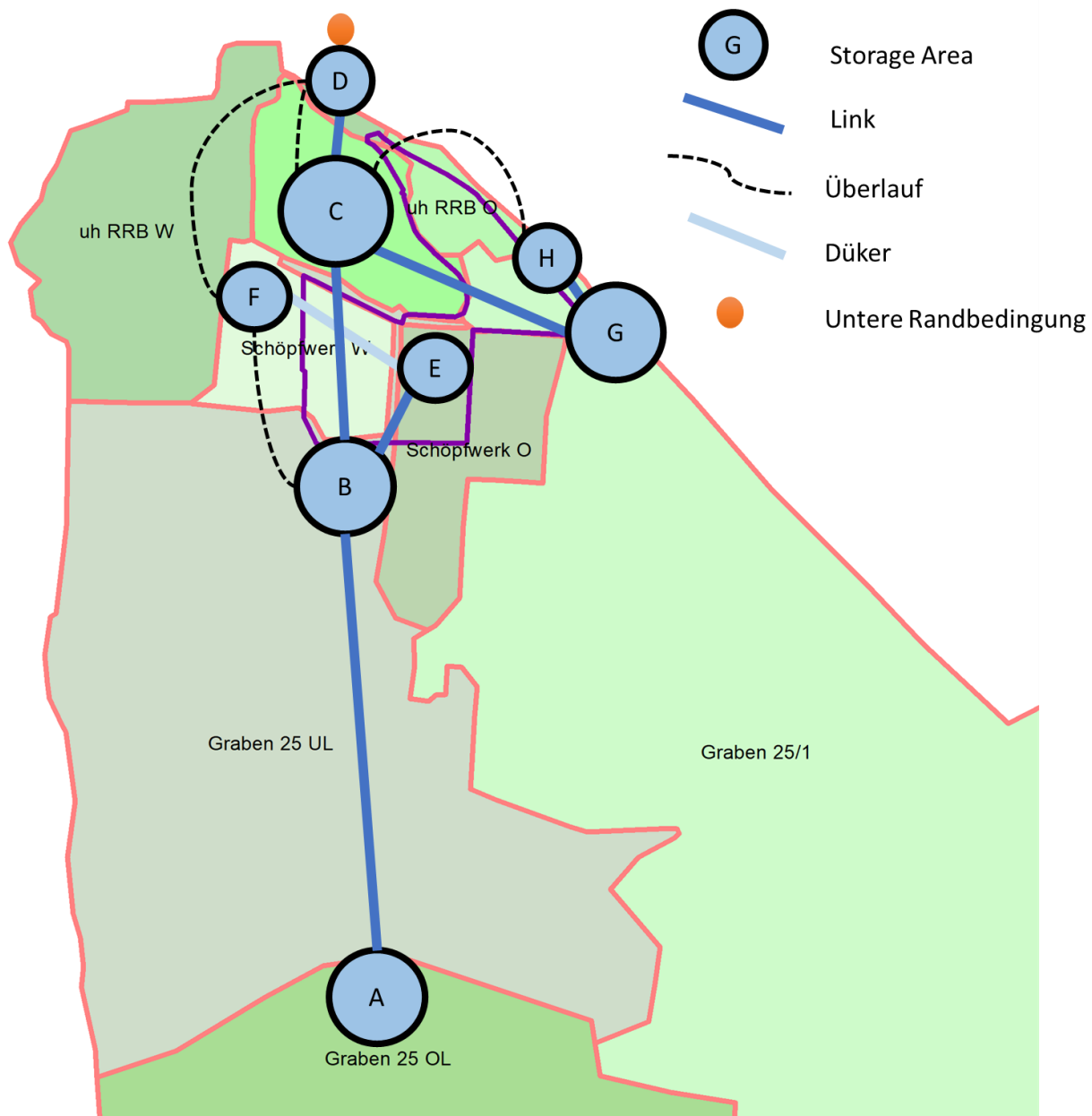
Abbildung 3-28: Modellierte Speicher (Storage Areas), Gewässerverbindungen (Links) und Wasserübertritte in Nachbargebiete im Extremfall (Überläufe)
