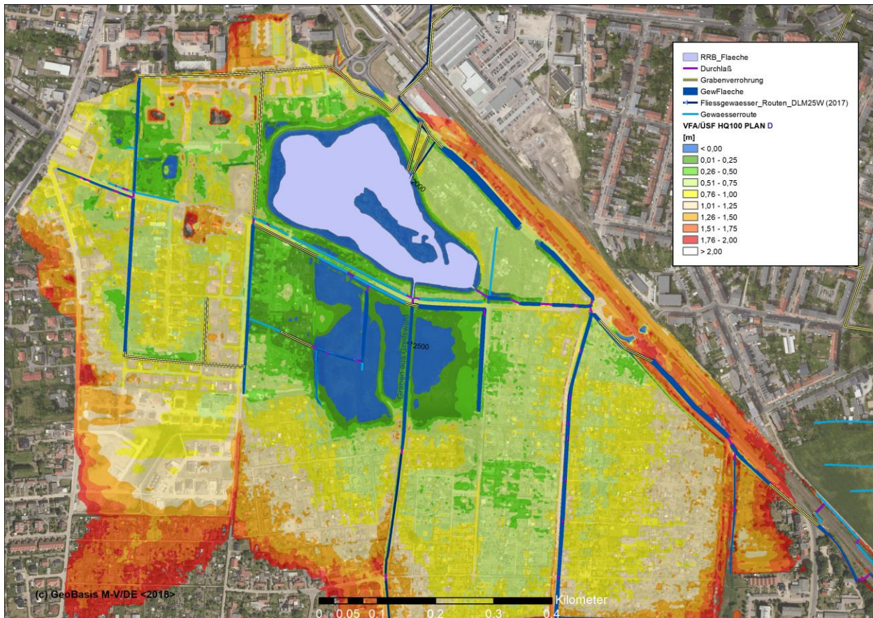
Abbildung 3-35: Vorflutabstände (grün-rot) / Überschwemmungsflächen (blau) bei HQ 100 im PLAN-D-Zustand
