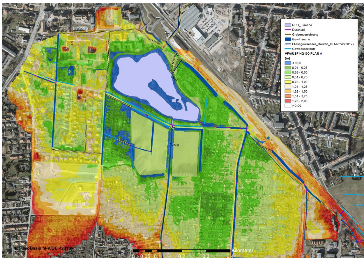
Abbildung 3-32: Vorflutabstände (grün-rot) / Überschwemmungsflächen (blau) bei HQ 100 im PLAN-A-Zustand
