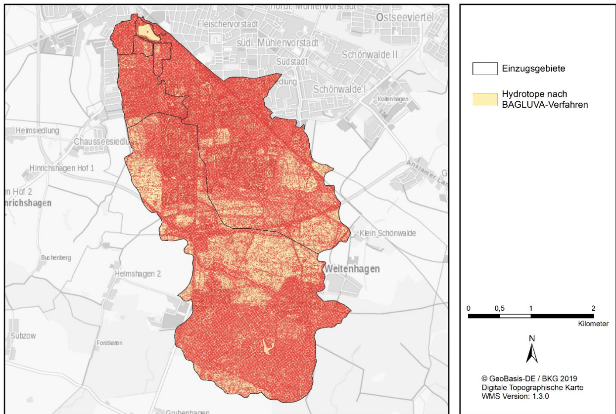
Abbildung 3-10: Im BAGLUVA-Verfahren definierte Hydrotöpfe im Untersuchungsgebiet
