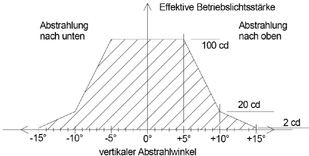
Abbildung 2 Vertikale Lichtstärkeverteilung Feuer W, rot
